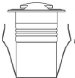
Ø52*H90mm
